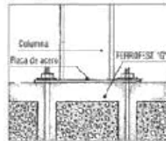
Fig. 4 ANCLAJE DE BARRAS Y PERNOS
