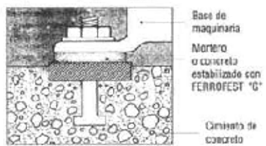
Fig. 3 ASENTAR MAQUINARIA
