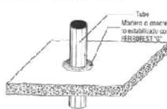
Fig. 7 RECIBIR TUBERIA Y CASQUILLOS
