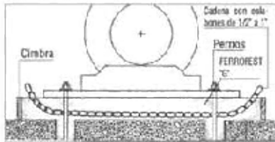
Fig. 3 ASENTAR MAQUINARIA
