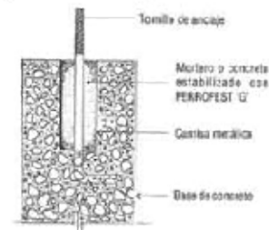
Fig. 8 RECIBIR ELEMENTOS
